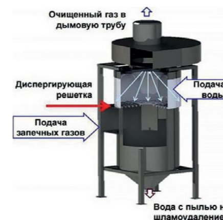
Газоочистное оборудование центробежно-вихревого типа
